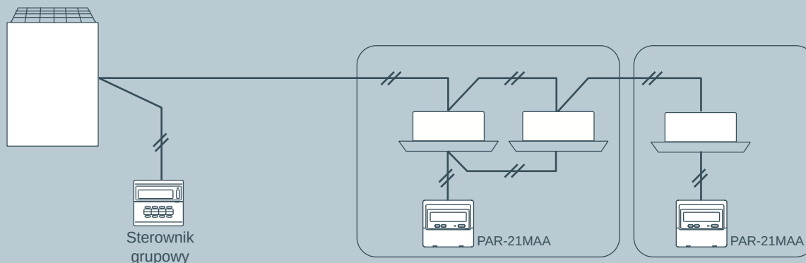
Połączenie z linią transmisji między jednostką wewnętrzną / zewnętrzną
