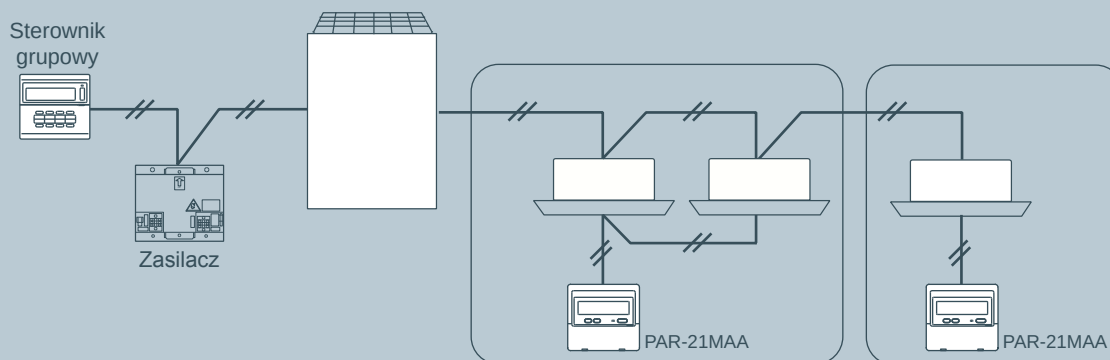
Połączenie z linią transmisji między jednostką wewnętrzną / zewnętrzną
